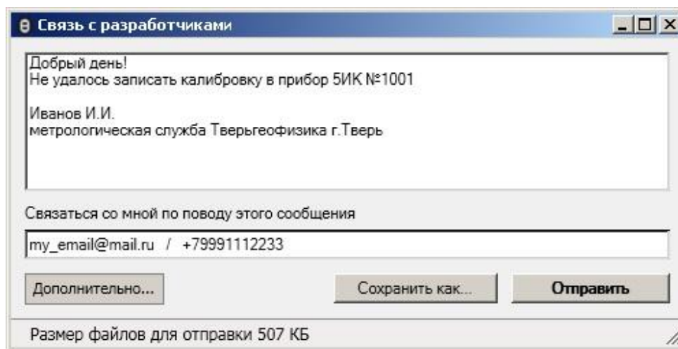
Рисунок 2.12.1 Формирование письма
