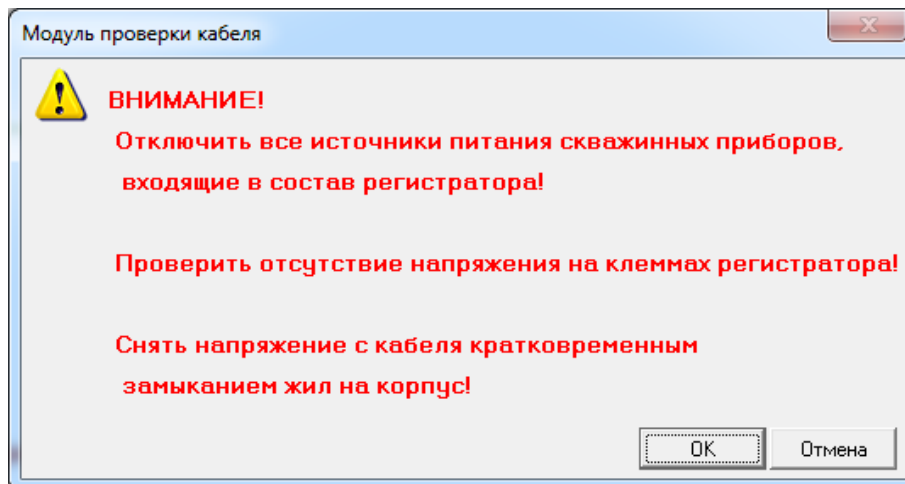
Рисунок 2.3.4.1 Окно предупреждения
