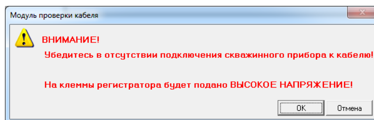
Рисунок 2.3.4.8 Окно предупреждения
