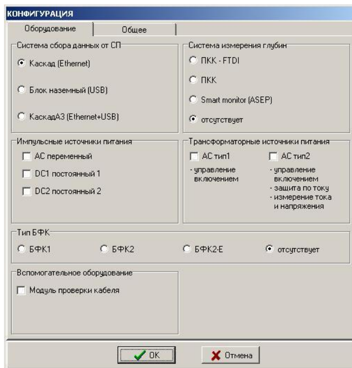
Рисунок 1.3.1 Окно «Конфигурация»
