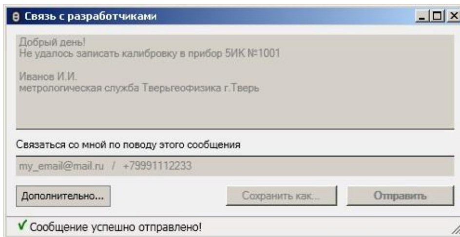
Рисунок 2.12.2 Отправка письма
